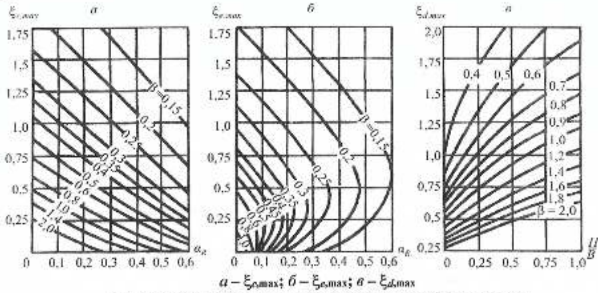
Рисунок К.3 – Графики для определения коэффициентов
