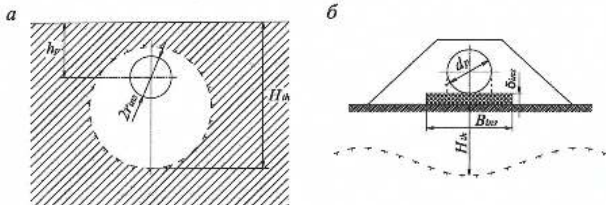
Рисунок Н.1 – Расчетная схема для определения глубины многолетнего оттаивания многолетнемерзлых грунтов под теплыми и горячими трубопроводами, проложенными подземно (а) и наземно (б)
