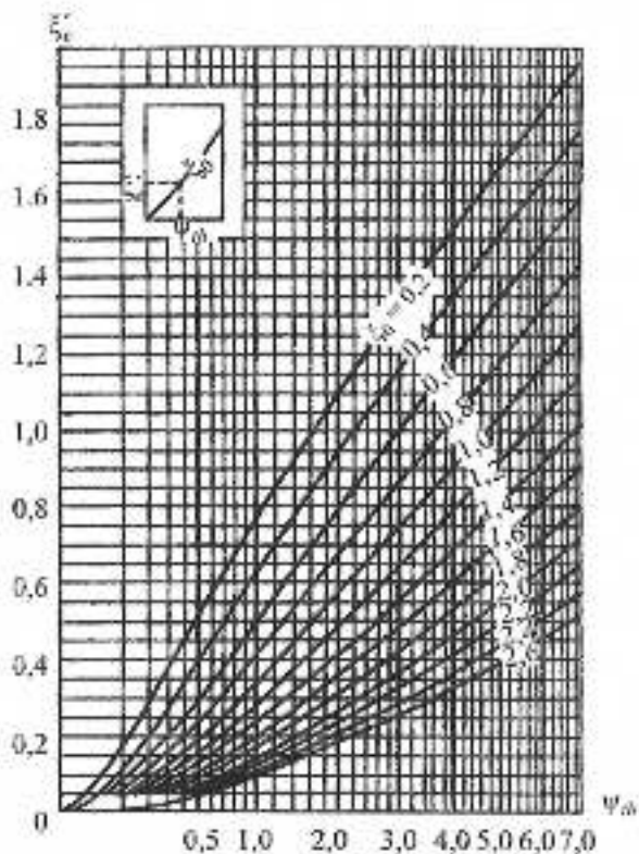
Рисунок К.6 – Графики для определения коэффициента \xi'_e
