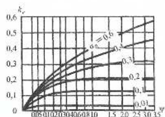
Рисунок К.2 – Графики для определения коэффициентов \xi_v и k_e
